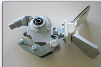
Doppel-Dosierperlpistole
