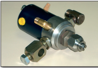
Пистолет-краскораспылитель Vialine Airless
