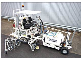
H18 Royal Air Force/Velká Británie, stroj pro značení 1K barvami za studena systémem Airless (dvě pumpy), značkovací jednotka pro značení šířky čáry 90 cm se 4 barvovými a 4 perlovými pistolemi a 3 barvovými a 3 perlovými pistolemi pro značení pruhu pro „taxi“ v barvách černá/žlutá/černá, tlakový zásobník o objemu 2 x 225 l
