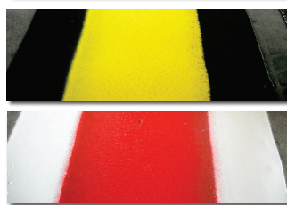
... für den Einsatz mit 90 cm Breitstrichmarkeur mit 4 Farbpistolen sowie weiteren 12 Farbpistolen für die Farben: weiß, rot, blau, gelb und schwarz, für „taxiways“ und Trennsicherheitslinien
