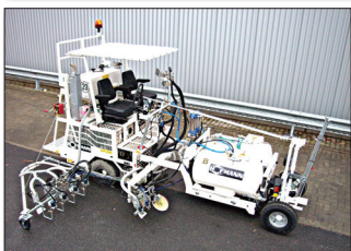
H18 bei Royal Air Force/UK mit 1K Kaltfarben Airless System (zwei Pumpen) für den Einsatz mit 90 cm Breitstrichmarkeur mit 4 Farb- und Perlpietolen sowie 3 Farb- und Perlpietolen für „taxiways“ in schwarz/gelb/schwarz, 2 x 225 ltr Druckbehälter
