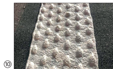
Marquage MultiDotLine®Plus, marquage profilé sur marquage pleins en un passage.
